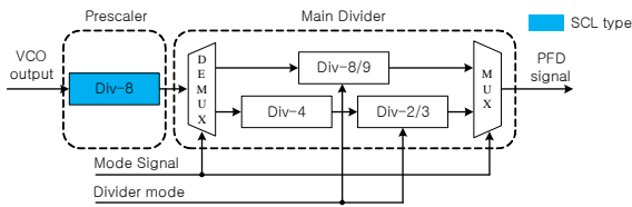
그림 7. 전치분주기와 주분주기의 구조 Fig. 7. Architecture of the prescaler and main divider.
