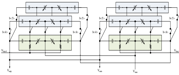
그림 3. 버랙터 뱅크의 구조 Fig. 3. Architecture of the varactor banks.
